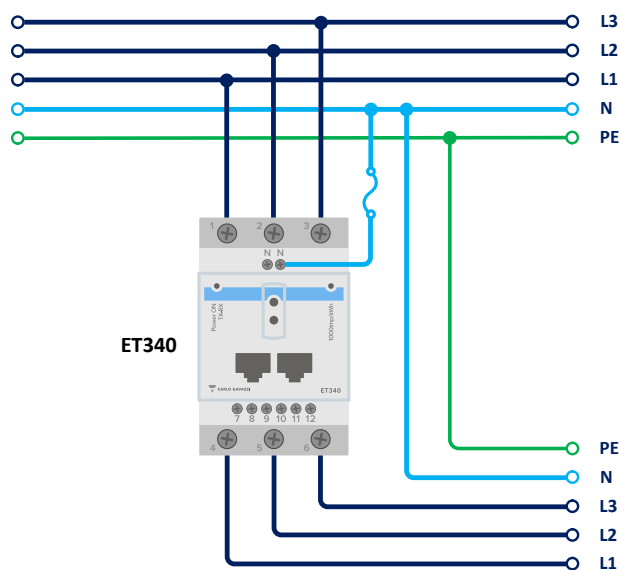
Cableado trifásico
